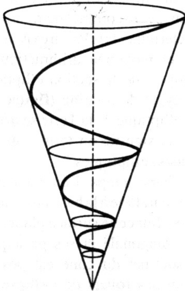
Figure 2. Une spirale logarithmique sur un cône.
